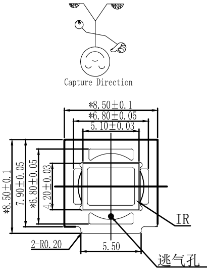
正面视图
