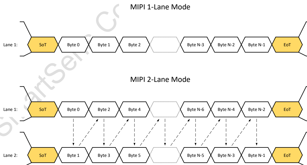
图 1-9 MIPI 1/2lane 模式数据包传输示意图
