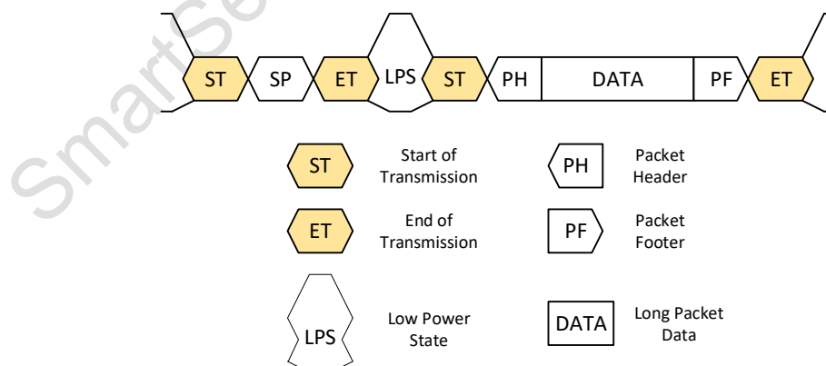
图 1-7 MIPI 底层数据包示意图
