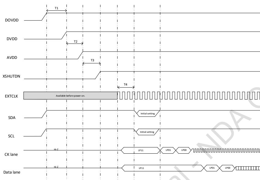
图 1-4 上电时序图
