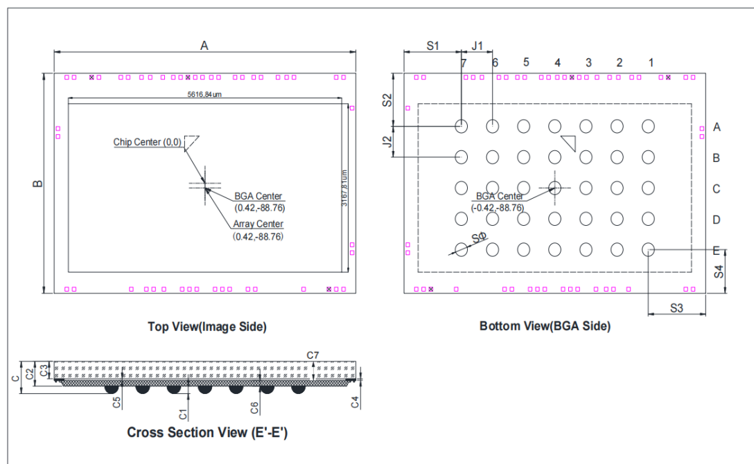
图 5-1 封装示意图
